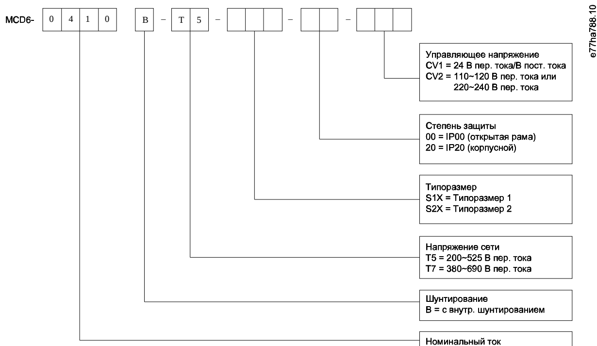
Рисунок 1: Строка кода типа
