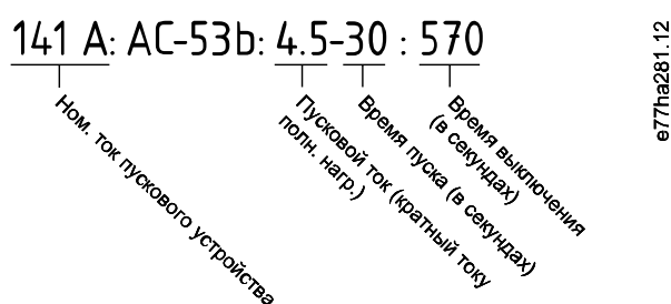
Рисунок 2: Формат AC53b
