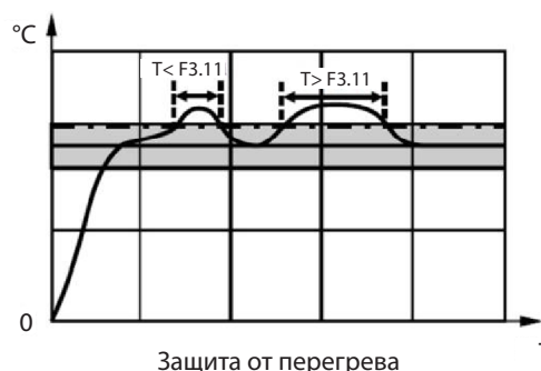
Защита от перегрева
