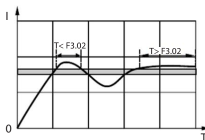
Характеристика защиты от перегрузки по току
